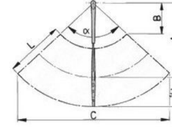
Одиночный поводок, регулируемый от 473 до 542
