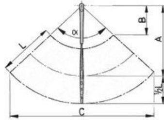
Одиночный поводок, регулируемый от 280 до 366
